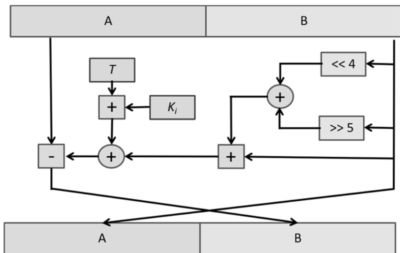
Рис. 3. Схема шифрування
